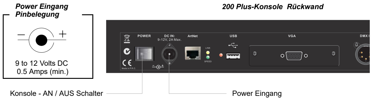
Abbildung 5: 200 Plus-Konsole Power-Anschluss
